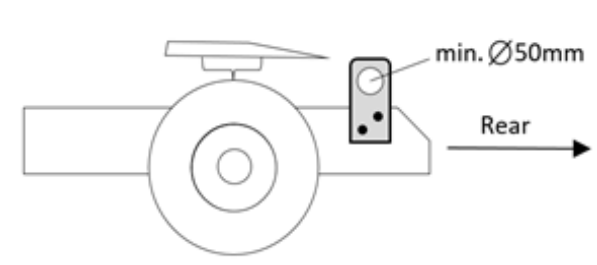
Dessin / Drawing 290-2.11.2
