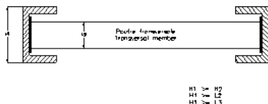
Dessin / Drawing 290-3.4.2
