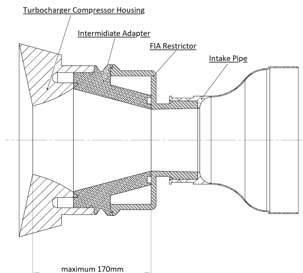
Dessin / Drawing 290-3.10.3
